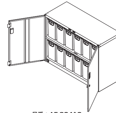
品番：AF-S0412 ・扉付きタイプ ・ファイルボックス小×12個 ・カギ2本付
